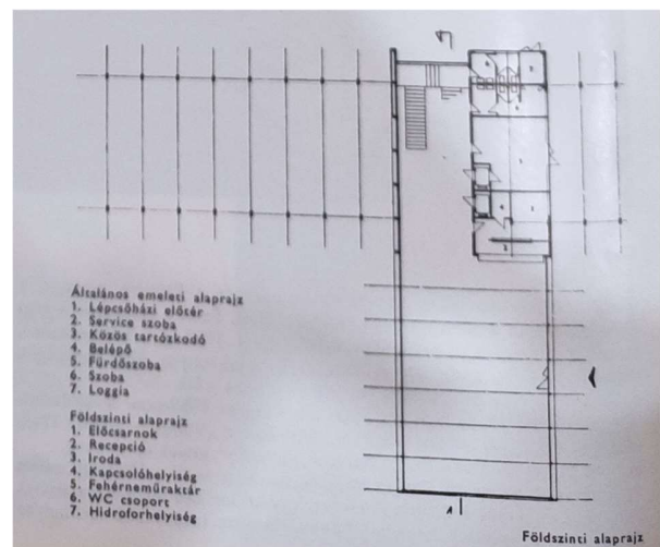
ábra 5.2.2. Balaton szálló földszinti alaprajz
