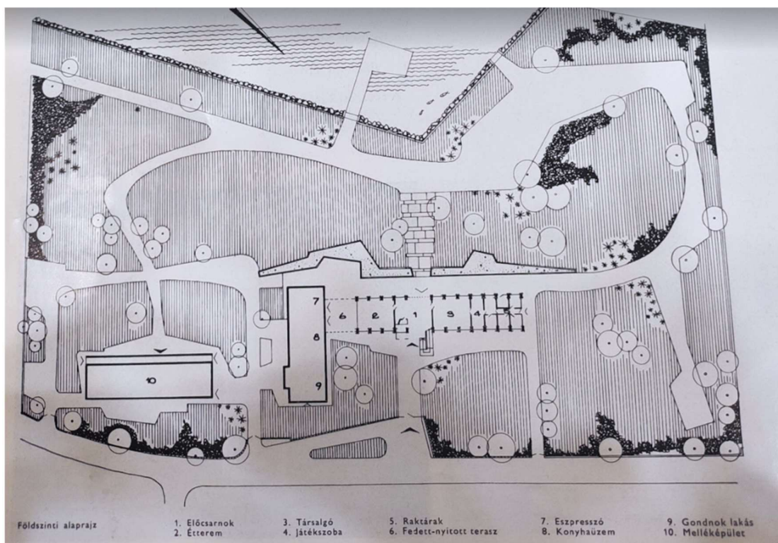
ábra 5.4.1. Kísérleti paneles idényszálló földszinti alaprajza, Balatonkenese
