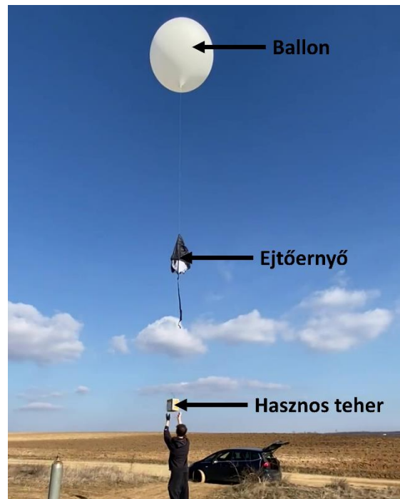
10. ábra – Az eszköz felépítése
