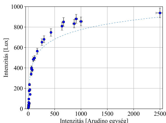
Fig. 4: Ezen az ábrán látható a fotoellenállás logaritmikus függése a valódi fényintenzitástól.
