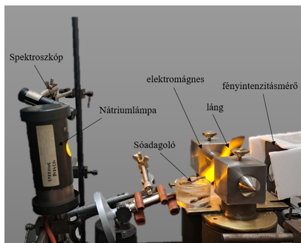
Fig. 3: A mérési elrendezés. Megfigyelhető, hogy a láng körül egy fekete szegély alakul ki a nátriumlámpa fényében.
