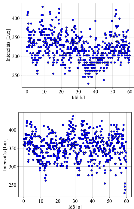
Fig. 5: A felső grafikonon ábrázolja azt az esetet, amikor a mágneses mező nem aktív, az alsó pedig egy 0.2T mágneses mezőben készült méréseket ábrázolja.
