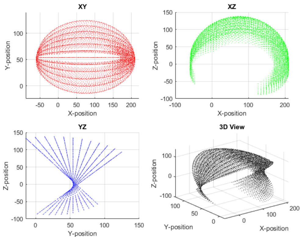
10. ábra. Egy láb munkatere MATLAB segítségével generálva.
