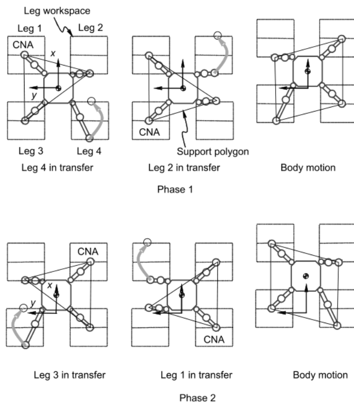
21. ábra. Két fázisú szaggatott járás szekvenciája [6].
