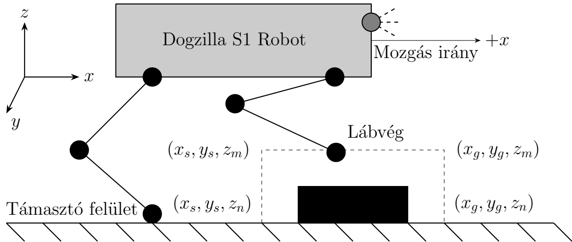
18. ábra. Lépésfüggvény meghatározása akár akadálykerülés céljából, 2-dimenzióra leegyszerűsítve.
