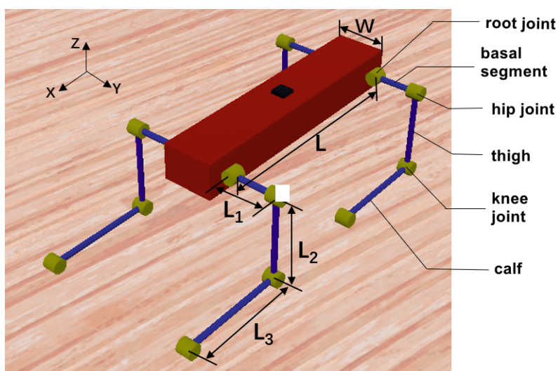
9. ábra. Dogzilla S1 egyszerűsített modellje Webots szimulációs környezetben [15].
