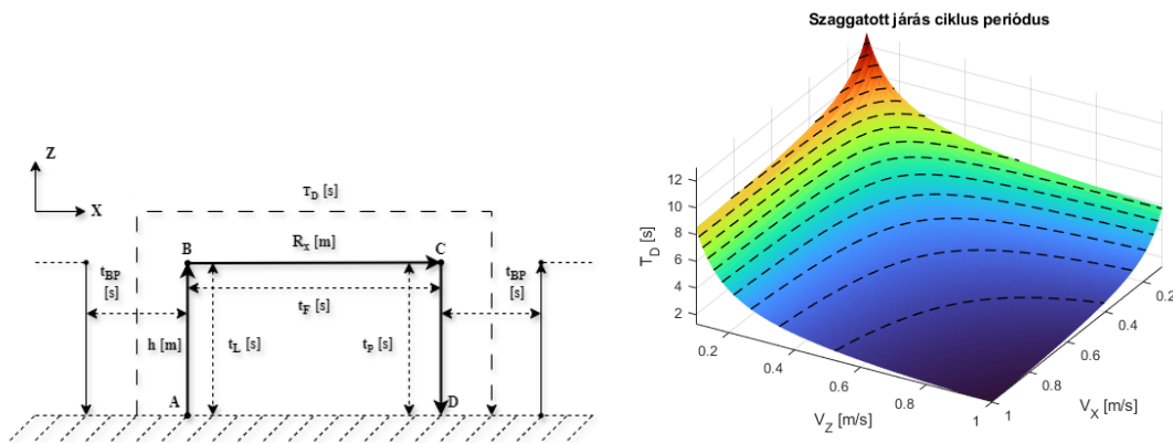
14. ábra. Szaggatott járás periódusa.
