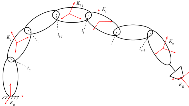
3. ábra. Egy robot manipulátor elvi rajza [8].
