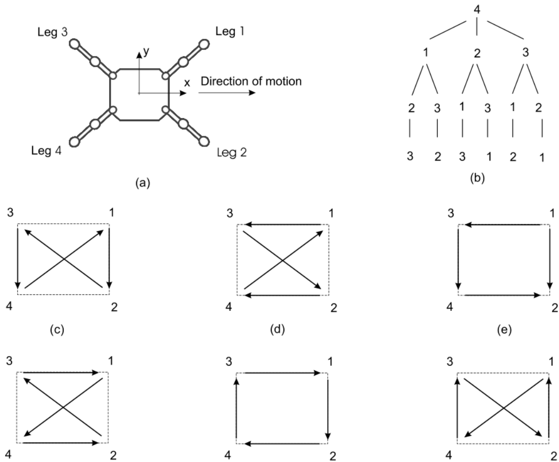
11. ábra. Lehetséges lépés esemény-szekvencia egy négylábú robot esetében [6].
