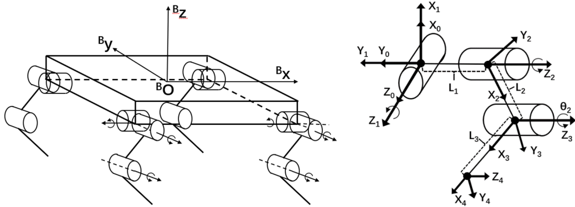
8. ábra. Robot koordináta-rendszerei. [15]
