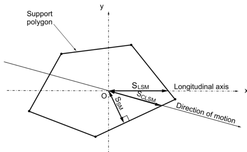
5. ábra. Támasztó-poligon és különböző stabilitási határok [6].
