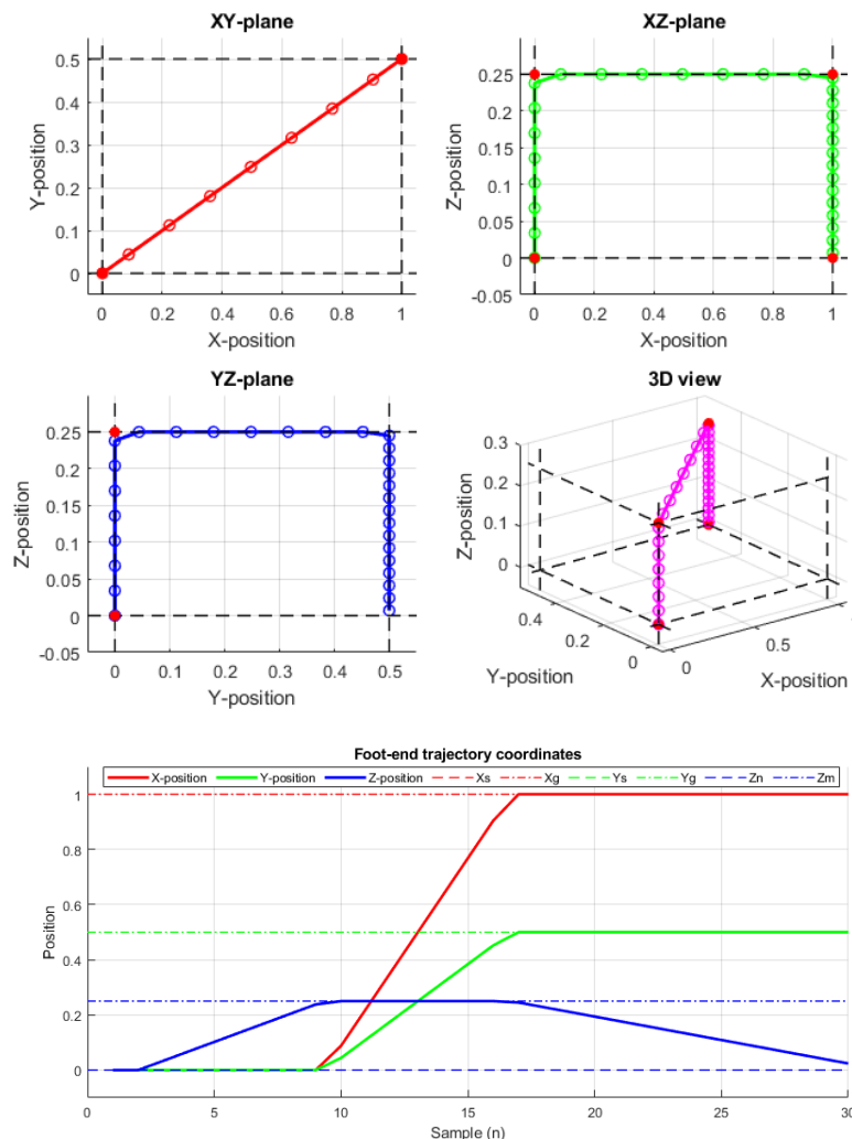
19. ábra. Lábvég pályájának generálása MATLAB környezetben.
