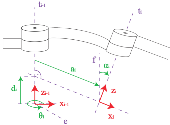
4. ábra. Denavit-Hartenberg paraméterek [8].
