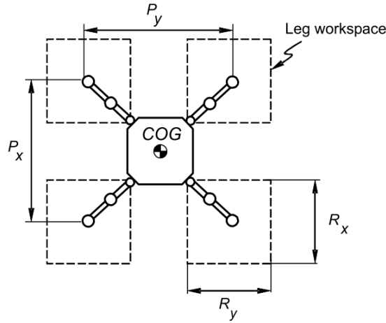
12. ábra. Lépés geometriai meghatározása [6].
