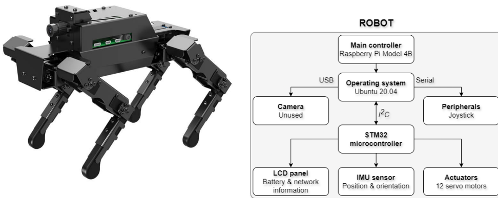
6. ábra. Dogzilla S1 Robotkutya és architektúrája [14]
