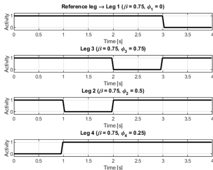
20. ábra. Eseményszekvencia tervezése.
