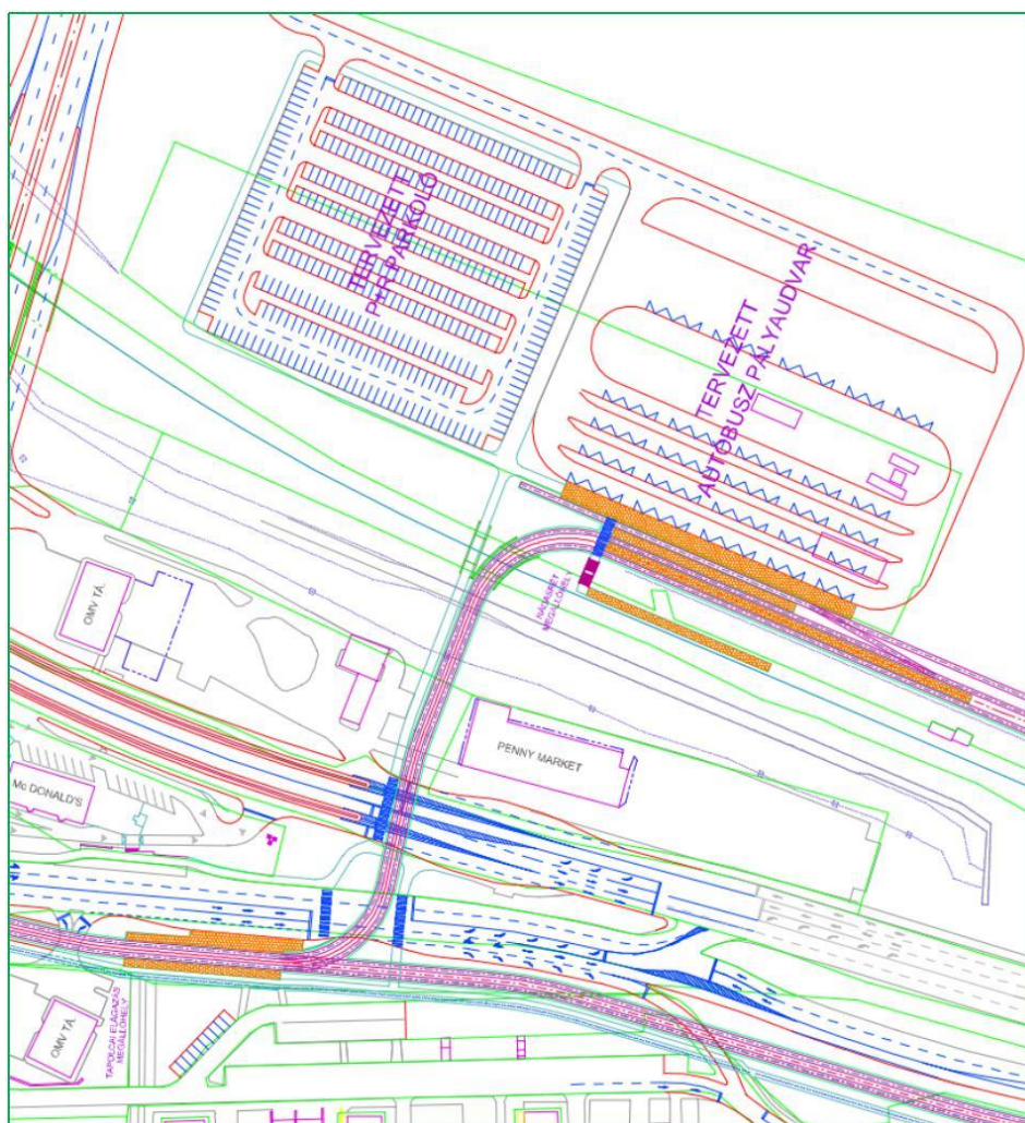
18. ábra: A Tapolcai elágazás villamos-megállóhely és a Tapolcai elágazás / Nadasrét villamos-végállomás egy korábban készült tervrajzon, helyi autóbusz-végállomással és P+R parkolóval (forrás: Szolgáltatói javaslatok a Miskolc, észak–déli villamosvonal tanulmánytervéhez. MVK Zrt., 2022)
