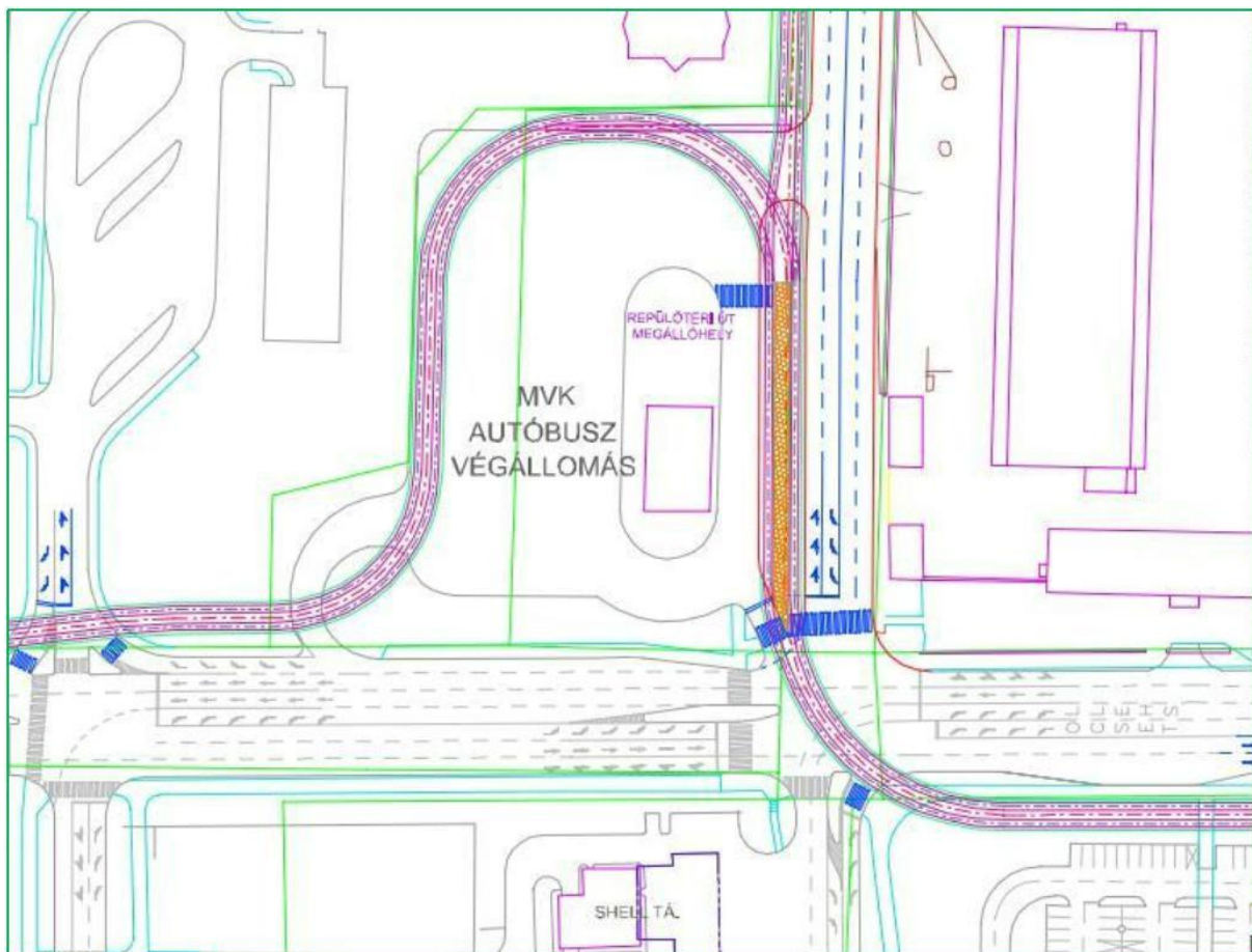
11. ábra: Az É-D-i villamosvonal repülőtéri elágazásánál lévő végállomásának vázlatrajza (forrás: Szolgáltatói javaslatok a Miskolc, észak–déli villamosvonal tanulmánytervéhez. MVK Zrt., 2022)
