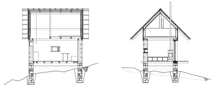
52.Kép: Metszetek - Kísérleti házikó, Sepsibesenyő [25]
