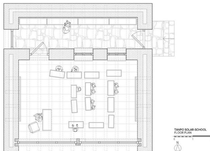
54.Kép: Napiskola, Tanpo - Alaprajz [26]
