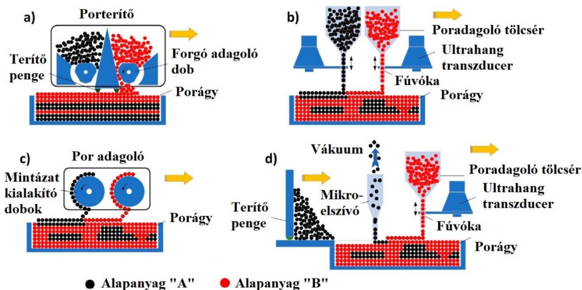
9. ábra Két alapanyagú poradagoló berendezések ábrái: a) Penge-alapú porteritő, b) Ultrahang alapú porteritő, c) Elektrofotografikus alapú porteritő, d) Penge és ultrahang alapú hibrid porteritő rendszerek [19]
