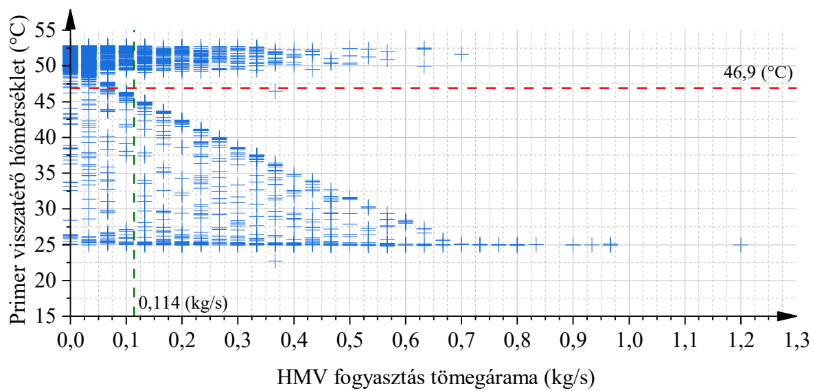
5. M-ábra, A v3 kapcsolás a II. esetben
