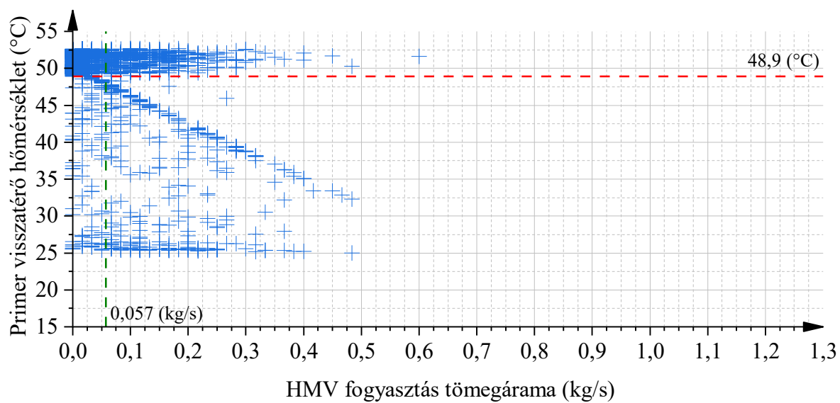
6. M-ábra, A v3 kapcsolás a III. esetben
