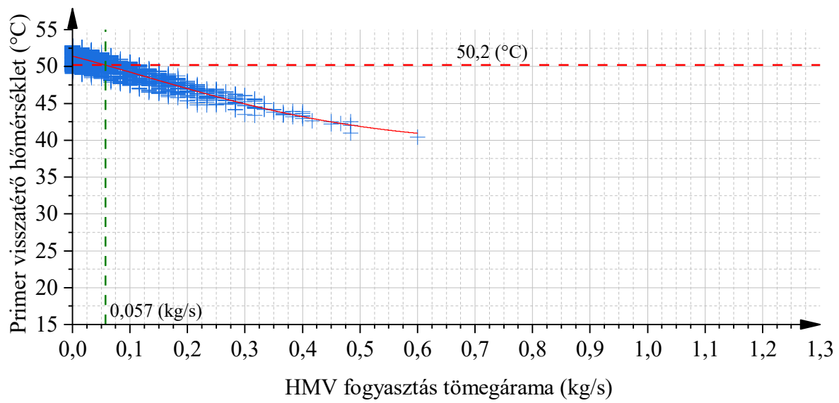
3. M-ábra, A v2 kapcsolás az I. esetben
