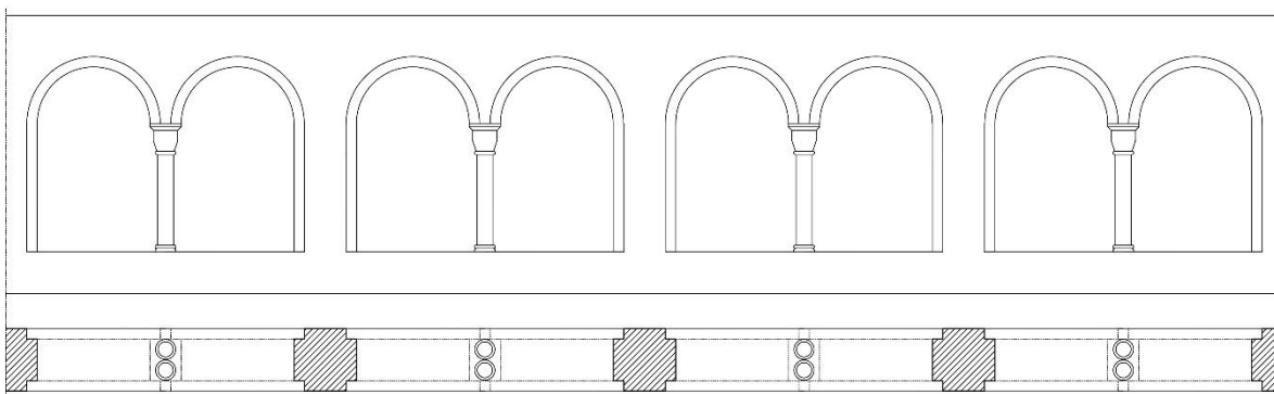
10. ábra A kerengő homlokzati kiosztása, 2024 (saját rajz)
