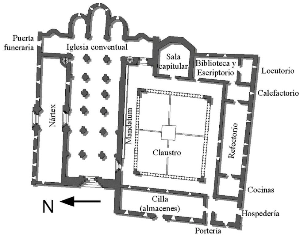
10. ábra: Santo Domingo de Silos alaprajza
