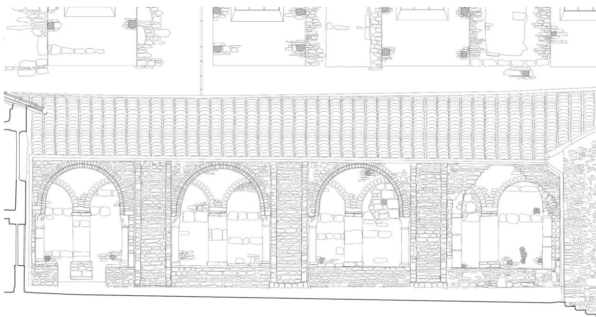
32. ábra: BME Építészettörténeti és Műemléki tanszék felmérőtábor: Az északi kerengő külső oldala, 1:50, 2023. (BME Építészettörténeti és Műemléki Tanszék)
