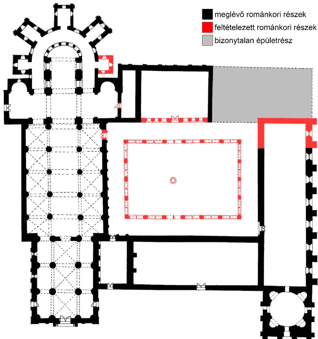
37. ábra: Az elméleti rekonstrukció alaprajza, 2024 (saját ábra)
