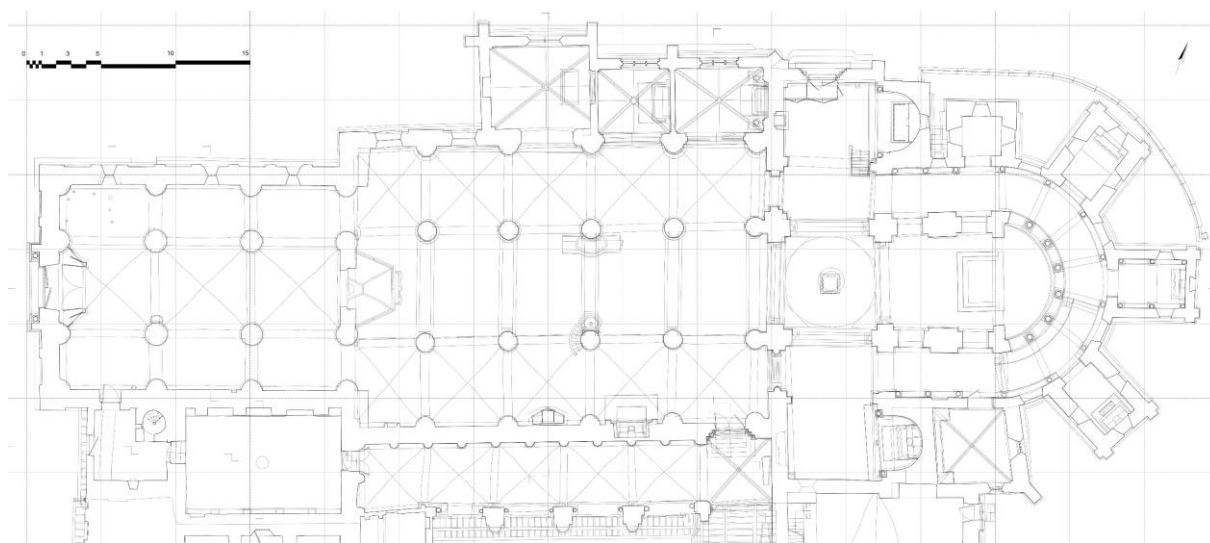
1. ábra: BME Építészettörténeti és Műemléki tanszék felmérőtábor: A Saint-Philibert templom alaprajza, 1:50, 2023. (BME Építészettörténeti és Műemléki Tanszék)
