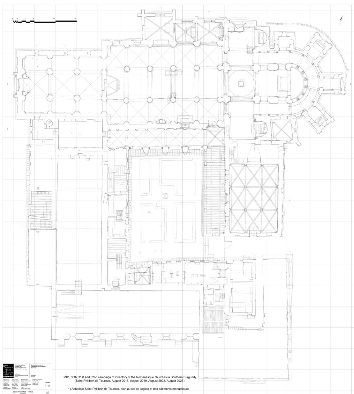
34. ábra: BME Építészettörténeti és Műemléki tanszék felmérőtábor: az együttes alaprajza, 1:50, 2023. (BME Építészettörténeti és Műemléki Tanszék)
