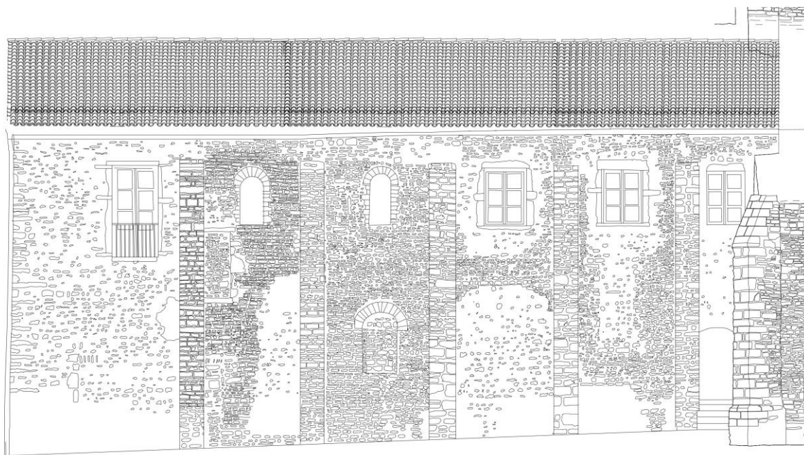
19. ábra: BME Építészettörténeti és Műemléki tanszék felmérőtábor: káptalanterem nyugati homlokzata, 1:50, 2023. (BME Építészettörténeti és Műemléki Tanszék)
