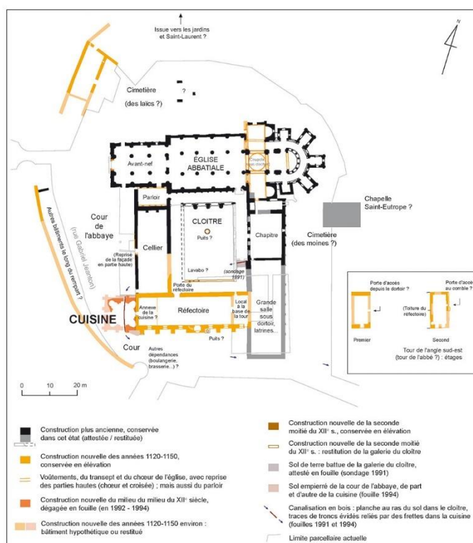
24. ábra (Saint-Jean-Vitus periodizációs alaprajza a 12.sz-i állapotáról ( https://books.openedition.org/artehis/5857 , utolsó látogatás: 2024.10.24.)
