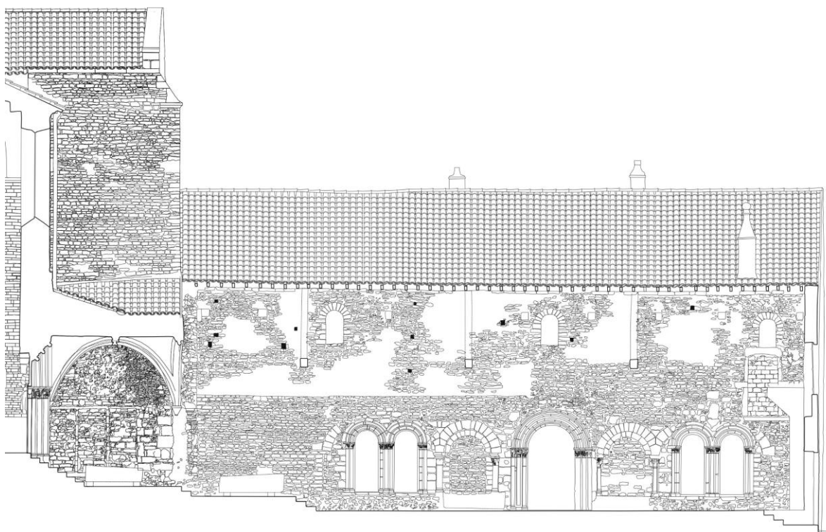
19. ábra: BME Építészettörténeti és Műemléki tanszék felmérőtábor: káptalanterem nyugati homlokzata, 1:50, 2023. (BME Építészettörténeti és Műemléki Tanszék)
