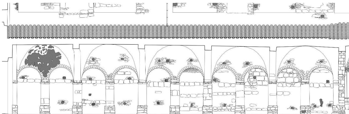
33. ábra: BME Építészettörténeti és Műemléki tanszék felmérőtábor: Az északi kerengő belső oldala, 1:50, 2023. (BME Építészettörténeti és Műemléki Tanszék)
