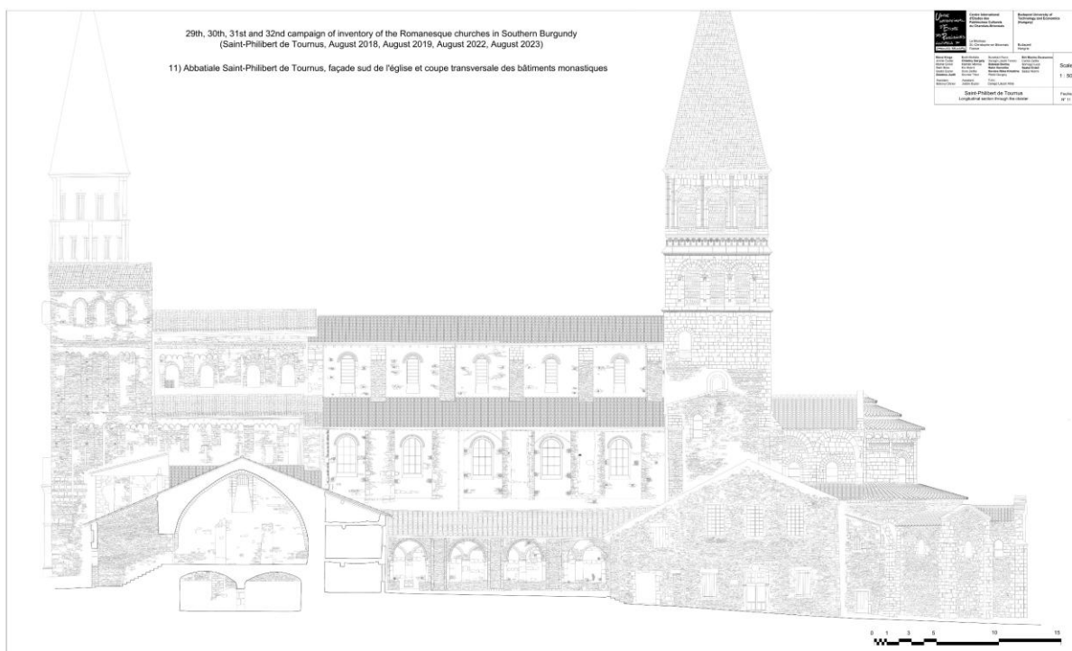
27. ábra: BME Építészettörténeti és Műemléki tanszék felmérőtábor: Az együttes metszete a nyugati szárnyon át észak felé, 1:50, 2023. (BME Építészettörténeti és Műemléki Tanszék)
