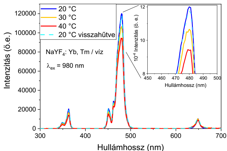
14. ábra: 1 mg/ml vizes UCNP-szuszpenzió emissziós spektruma különböző hőmérsékleteken 980 nm hullámhosszú lézergerjesztés mellett
