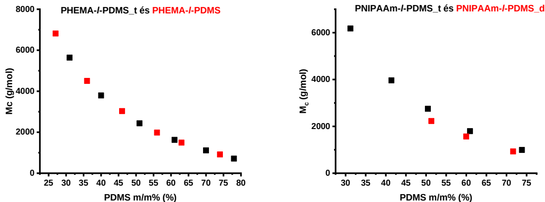
22. ábra. A polimer szegmensek keresztkötési pontok közötti átlagos molekulatömege ( M_c ) az összetétel szerint. Balra az PHEMA-I-PDMS I. (feketével) és II. (pirossal) sorozatának értékei, jobbra a PNIPAAm-I-PDMS III. (feketével) és IV. (pirossal) sorozatának értékei láthatók.
