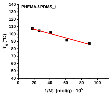
23. ábra. A PHEMA (balra) és PNIPAAm (jobbra) komponensek T_g -je az 1/M_c függvényében a PHEMA-I-PDMS és PNIPAAm-I-PDMS kotérhálókbán.
