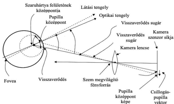
2. ábra: A PCCR módszer működési elve (Guestrin és M. Eizenman, 2006 alapján) [23]
