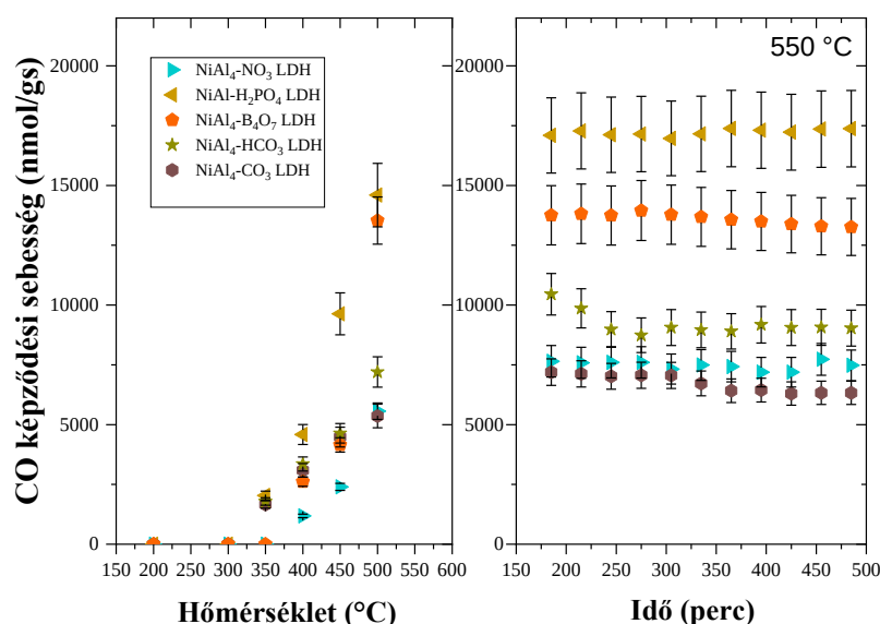
20. ábra: A CO képződési sebesség hőmérséklet (bal oldali) és idő (jobb oldali) függvényében a nitrát, a foszfor, a két szén, valamint a bór tartalmú katalizátorok esetén
