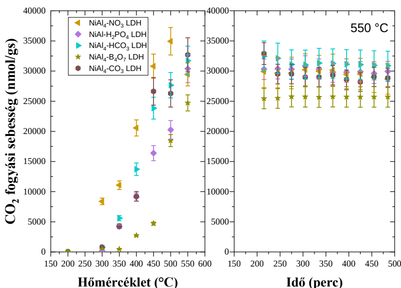
16. ábra: A \text{CO}_2 fogyasztási sebesség hőmérséklet (bal oldali) és idő (jobb oldali) függvényében a nitrát, a foszfor, a két szén, valamint a bór tartalmú katalizátorok esetén
