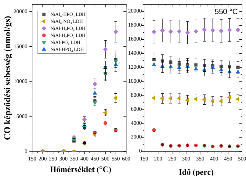
19. ábra: A CO képződési sebesség hőmérséklet (bal oldali) és idő (jobb oldali) függvényében az öt foszfor, valamint a nitrát tartalmú katalizátorok esetén
