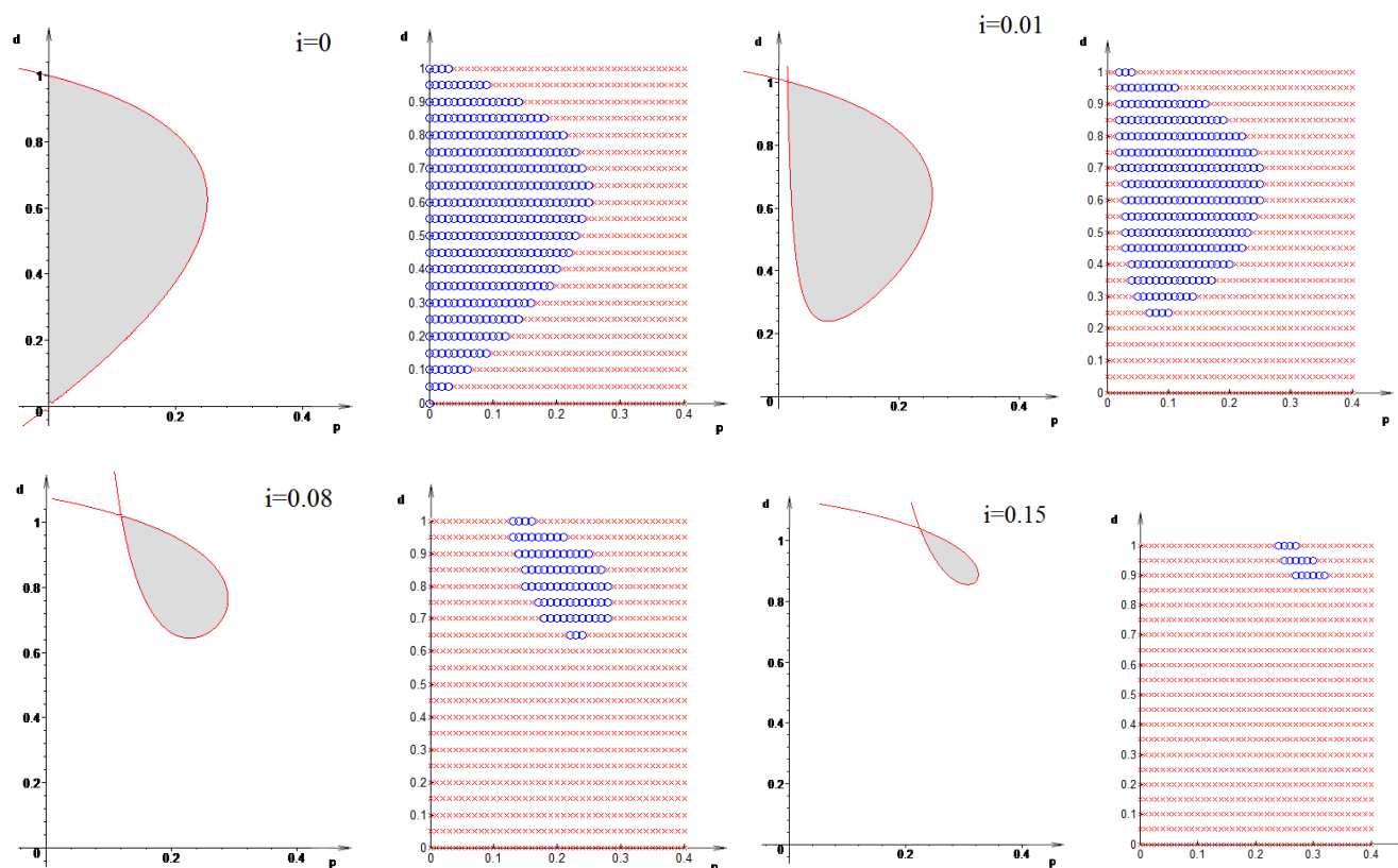
5-10. ábra A digitális PID szabályozás stabilitási térképe (A képpárok bal oldali eleme az analitikus megoldást mutatja, míg a képpárok jobboldali eleme a numerikus stabilitás vizsgálat eredményét, a szürke illetve a körökkel jelzett értékek jelzik a stabil paraméter kombinációkat)
