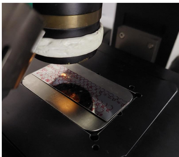
9. ábra: Polírozott acél tárgylemez kenetkezel a FT-IR spektrométer tárgyasztalán
