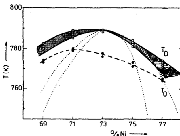
3. ábra. VAN DEEN & VAN DER WOUDE (1981) fázisdiagramja az awaruitról. „ T_D ” a rendezetlen fázist, „ T_O ” a rendezett fázist jelenti. A szürke zónában egyszerre van jelen a rendezett és a rendezetlen fázis.
