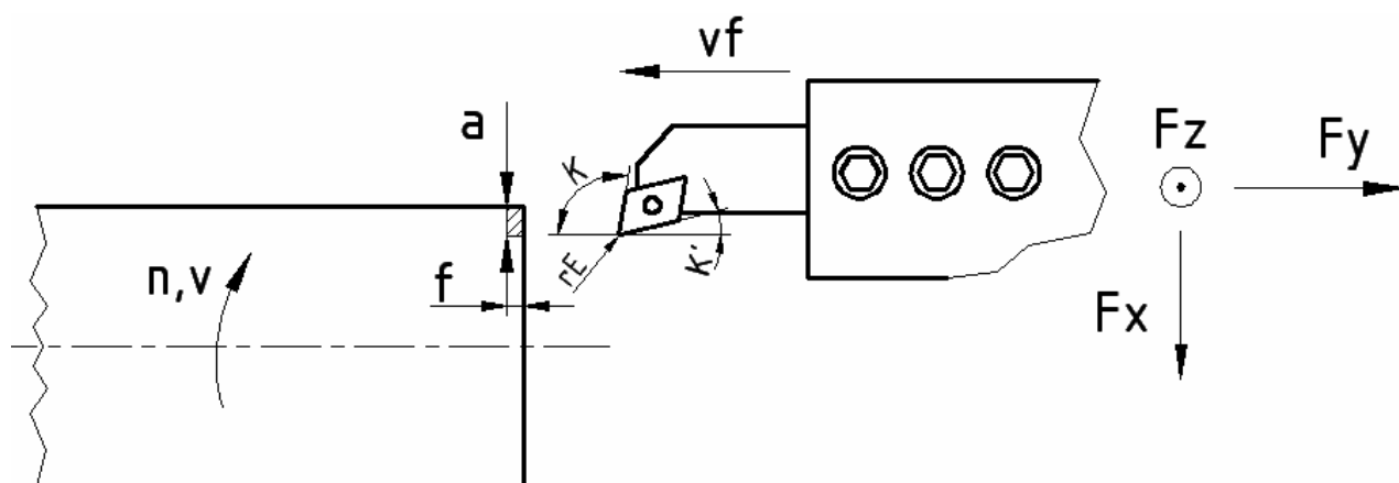
16.ábra. Hosszesztergálási mérési elrendezés
