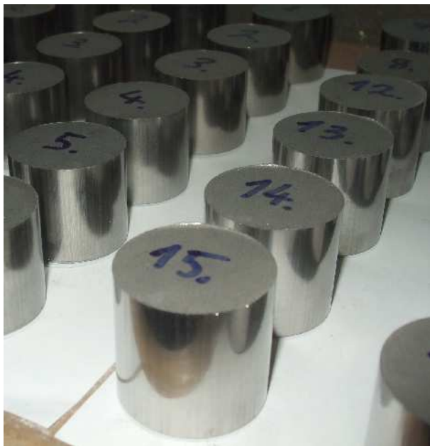
4. ábra. A sajtológépből kikerült próbatestek
