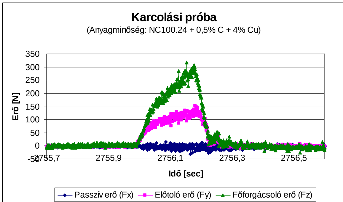
24.ábra. Karcolási próba során regisztrált spektrum
