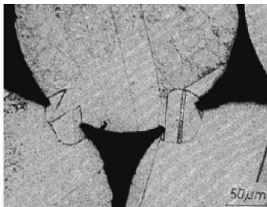
13.ábra. Nyakképződés a porszemcsék között
