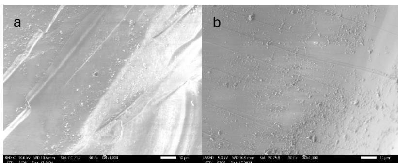
6. ábra Monoki vízopál (a) 10\text{kV} , 1000\times -es nagyítás (b) 5\text{kV} , 1000\times -es nagyítás
