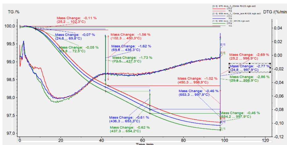
5. ábra Tömegvesztesség DTG görbe szerint a monoki vízipál esetében
