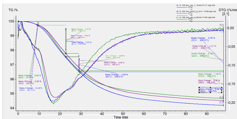
5. ábra Tömegveszteség DTG görbe szerint az erdőbényei viaszopál esetében
