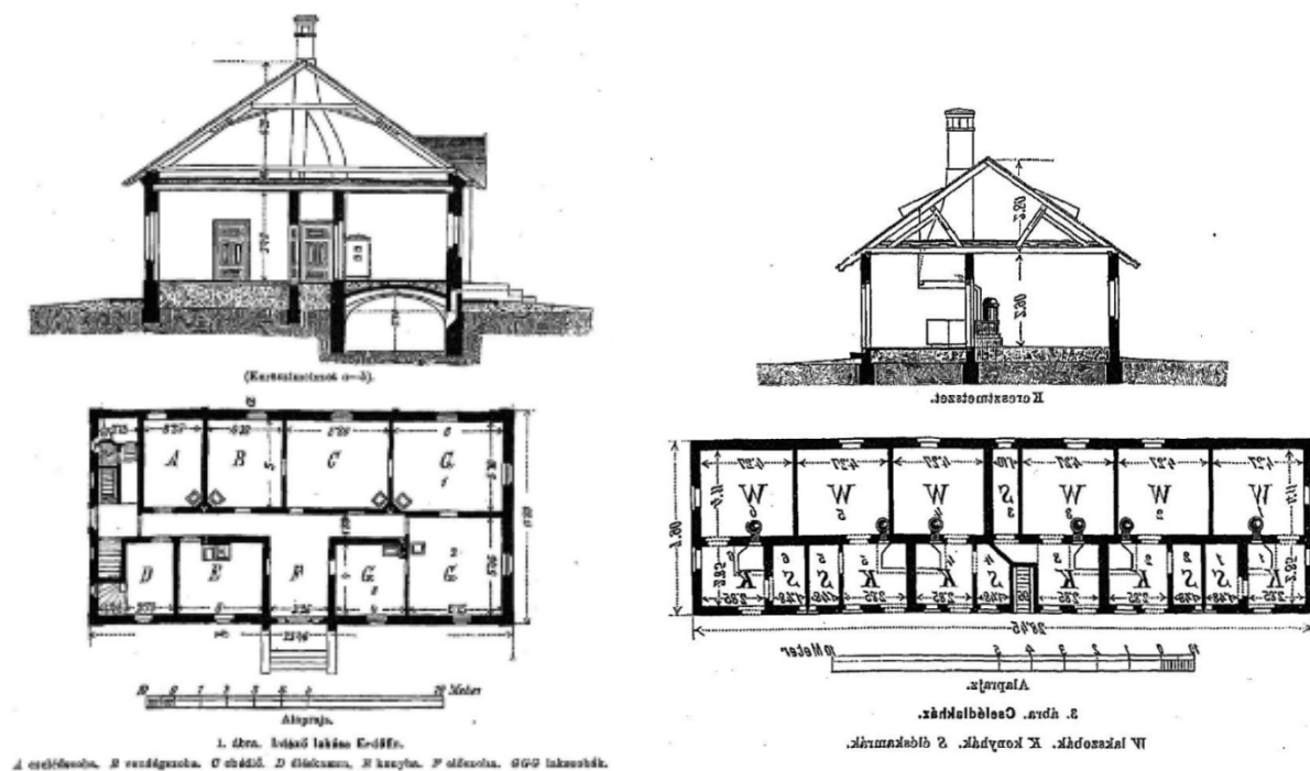
12. ábra: Az intézőház vagy kiskastély alaprajza és keresztmetszete balra, jobbra a cselédsor alaprajza és keresztmetszete.
