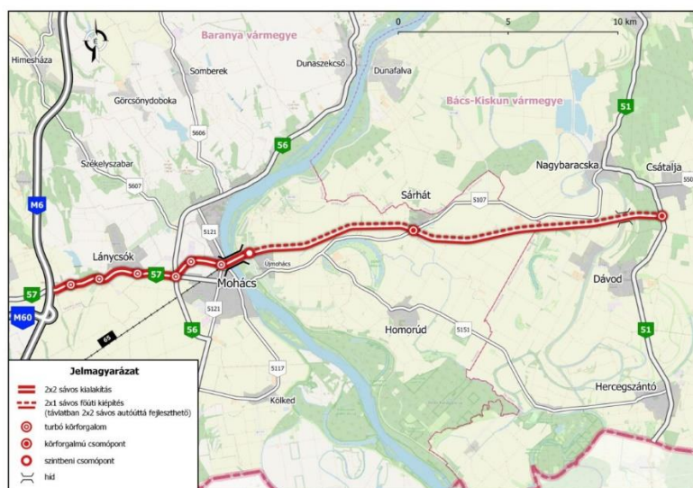
15. ábra: A híd tervezett nyomvonala.
