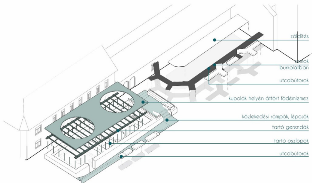
66. kép: koncepció robbantott ábrán
