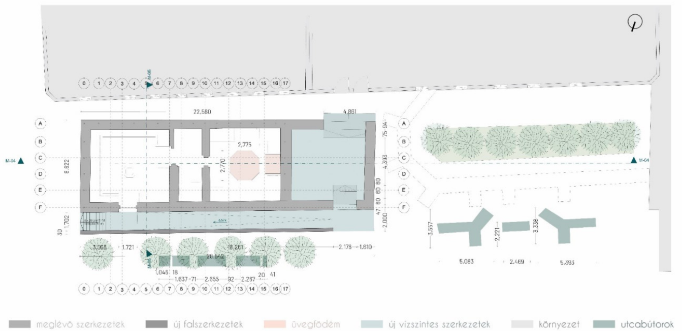
70. kép: vezérszinti alaprajz
