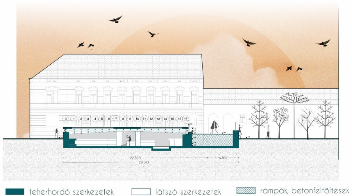
71. kép: M-04-hosszmetszet
