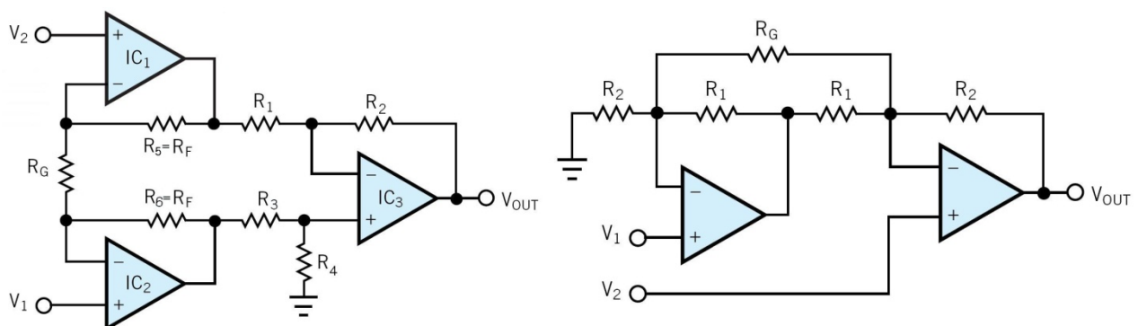
16. ábra: A 3- és 2 műveleti erősítős műszererősítők vázlatos felépítése [Man02]
