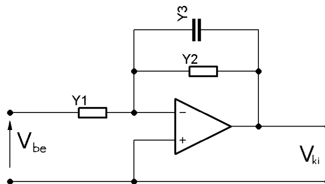
21. ábra: Az elsőrendű alul áteresztő szűrő impedancia modellje
