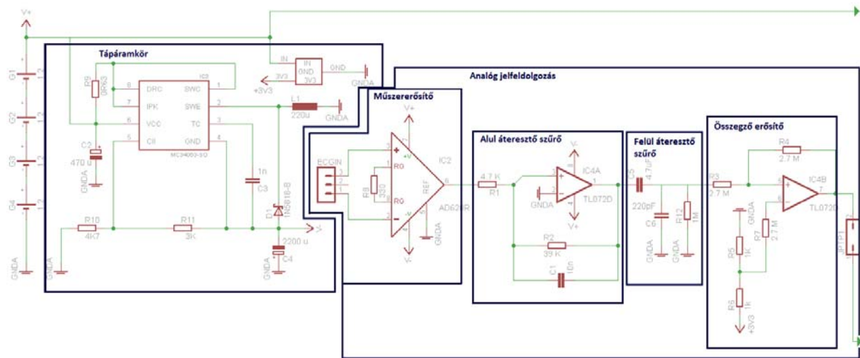
29. ábra: A feszültség invertáló és szabályozó tápfeszültség az analog jelfeldolgozó blokkal
