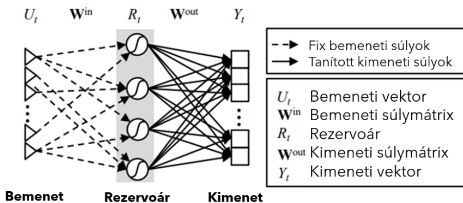
5. ábra. Egy rejtett réteggel rendelkező ELM illusztrációja. (Forrás: A. Jalvand, O. Asztalos, M. Karacsonyi and G. I. Pokol, "Application of neural networks in beam emission spectroscopy modelling" [28])
