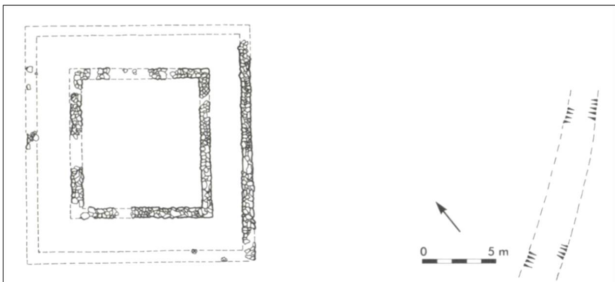
5. ábra: A Hatvan-Gombospusztán található burgus alaprajza. (Mráv 2003: 208.)
