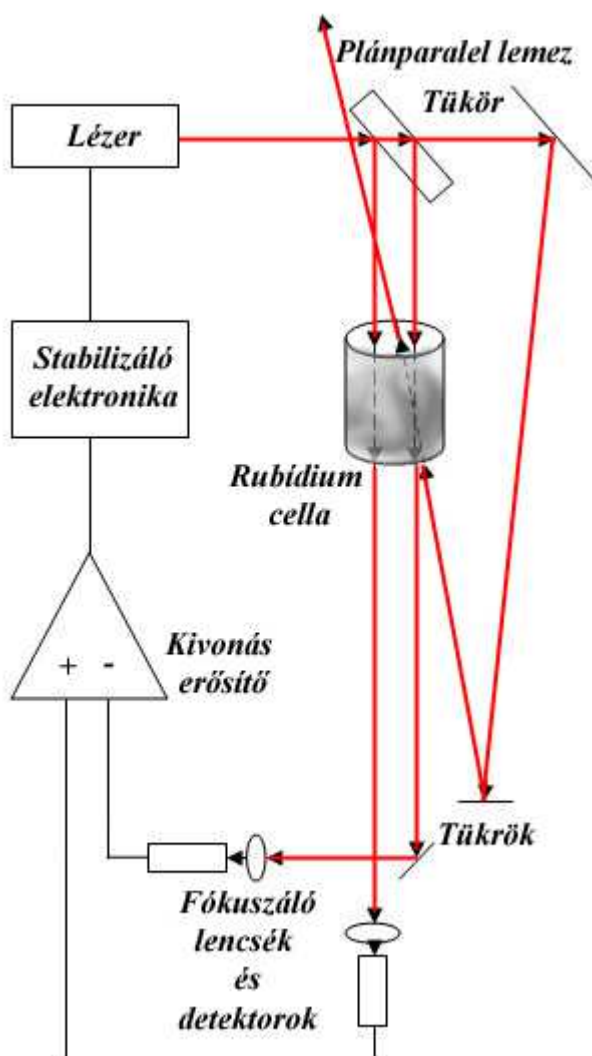
10. ábra - Telítési spektroszkópia mérési elrendezése
