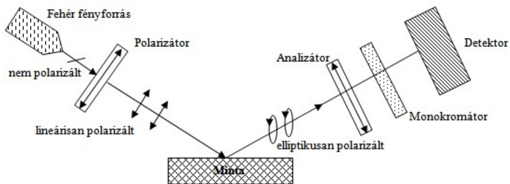
10. ábra: Ellipszométer elvi vázlata
