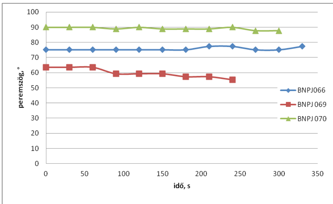
17. ábra – 60 mol% KI-KCl oldadék peremszögének változása az idő függvényében, grafit szubsztráton
