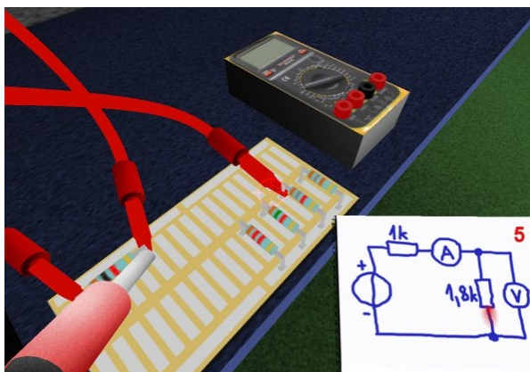
11. ábra: Ellenállás bekötése (Forrás: készítette Sátori László)
