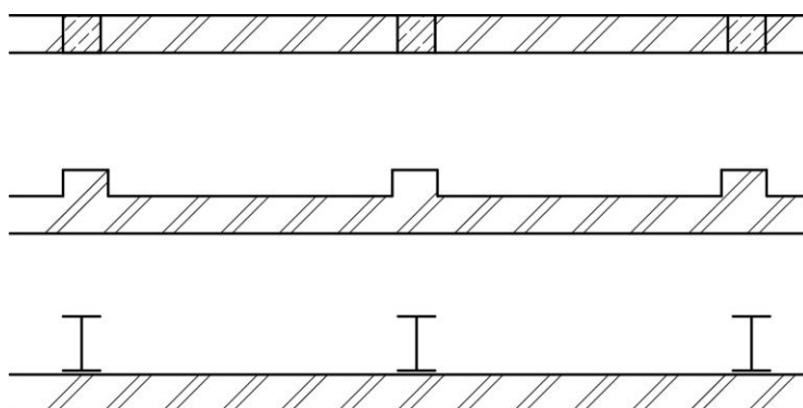
7.1. ábra: Falazat hosszának csökkentése függőleges bordákkal: vasbeton, falazott és acél pillér
