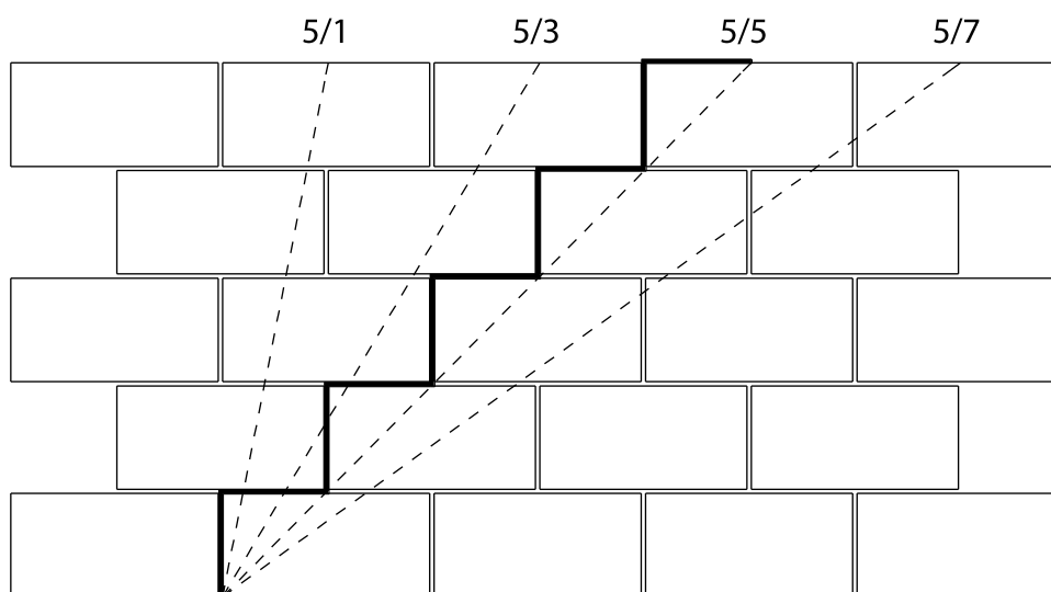
9.1 ábra: 5 téгла magas falon feltételezett törésvonal irányok
