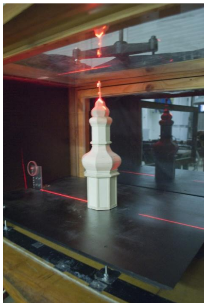
52. ábra A Tűztorony makettje a függőleges lézersíkkal megvilágítva a szélcsatorna mérőtérében
