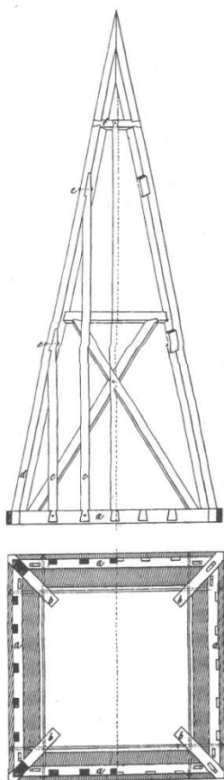
15. ábra Császárfás tetősisak a XVIII. században (forrás: Déry)
