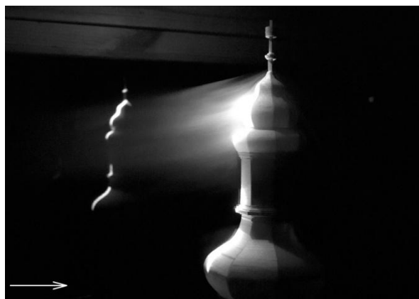
63. ábra A torony tetején az olajköd felkenődik az íveken
