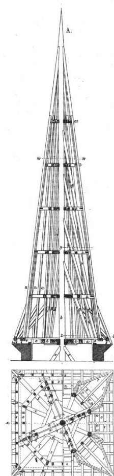
16. ábra Császárfás toronytető merevítőszintekkel (forrás: Déry)
