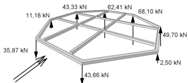
71. ábra Támaszerők önsúlya
