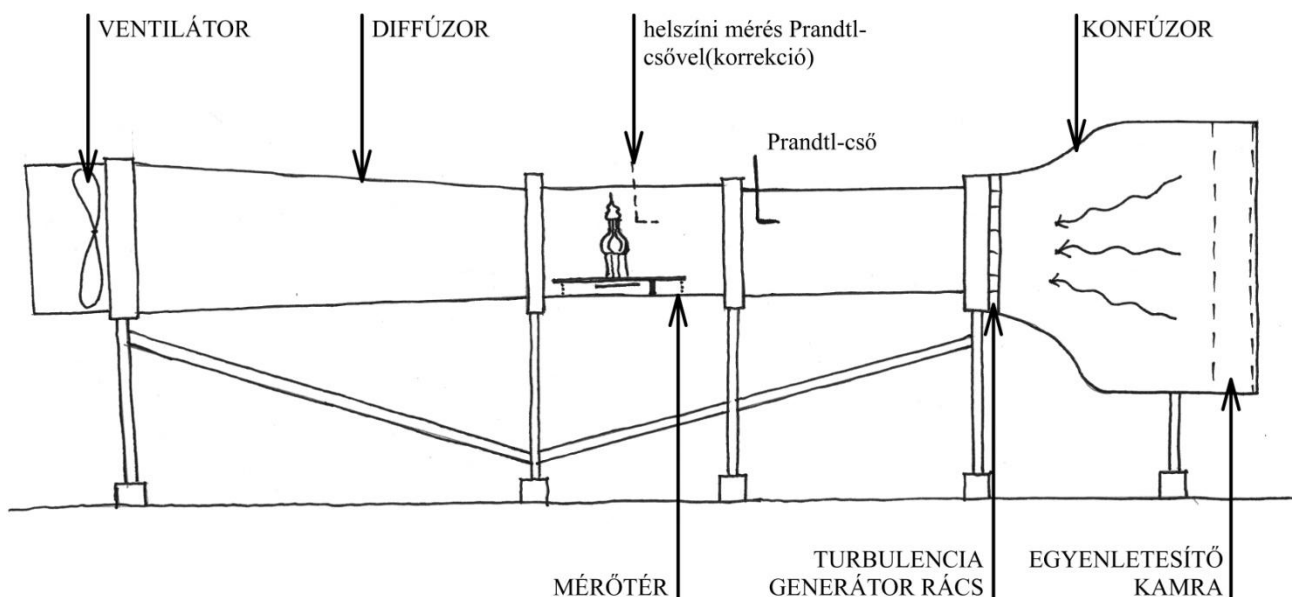
28. ábra Szélcsatorna rajza és működési elemei
