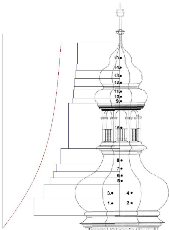
64. ábra q_p(z) torlónyomás profil (piros) és a terhelési mezők q_p(z_e) (kék) értékeinek viszonya
