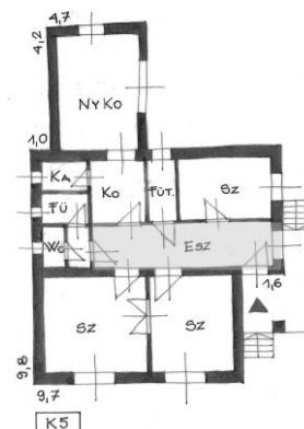
K5 zárt folyosója
