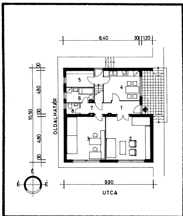
Sátortetős változat CS 00 H 13 AV S
