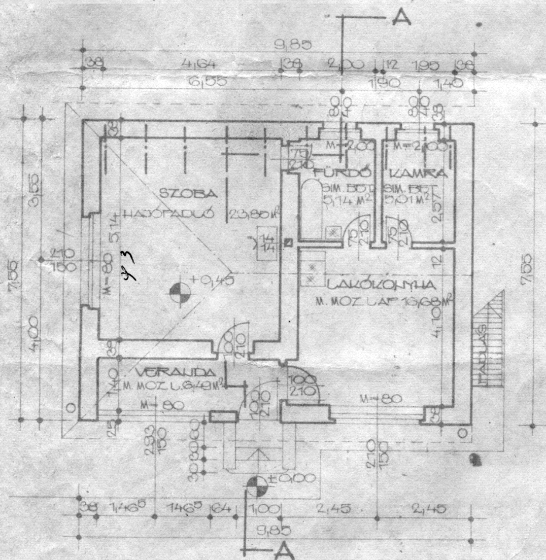
FÖLDSZINTI ALAPRAJZ
