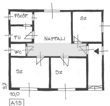
A13 nappali térré bővülő folyosója
