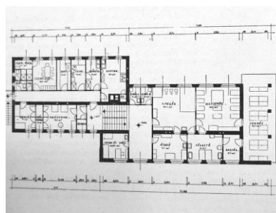
Bölcsőde típusúterve (Magyar Építőművészet 1956/4. )
