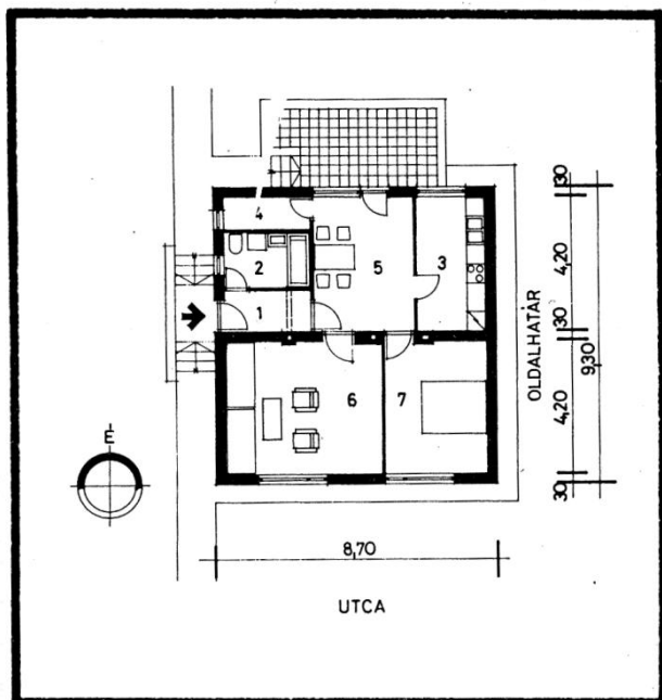
Sátortetős változat CS 00 H 21 A S
