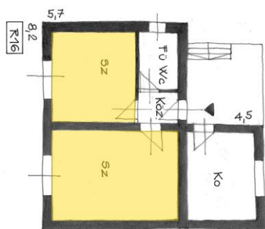
Rákóczi u. 16. utcafronti szobái
