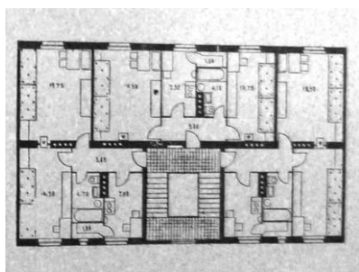
VÁTI típusúterv (Magyar Építőművészet 1952/6. )
