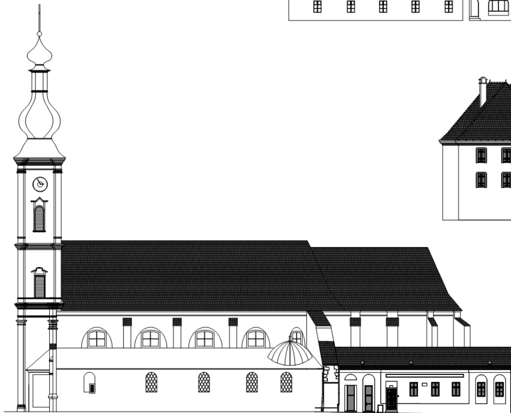
Déli homlokzat M1:300
