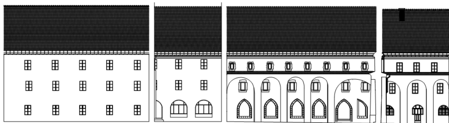
Kerengő homlokzatai M1:300
