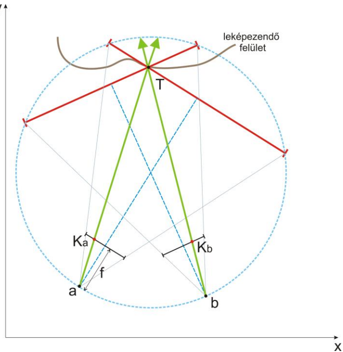
6. ábra: A képegyeztetés sematikus ábrája: A 2 kép vetítési centrumából az össze-tartozó homológ pontokon keresztül húzott egyenesek a térben a keresett felszíni pontban metsződnek.
