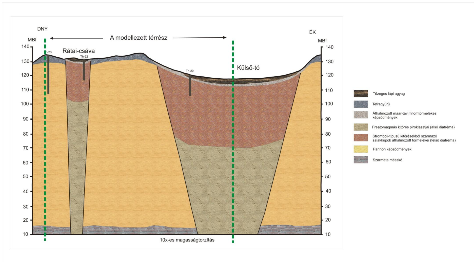
35. ábra: A Rátai-csáva és a Külső-tó között felvett szelvény, amely a numerikus modell alapját képezte
