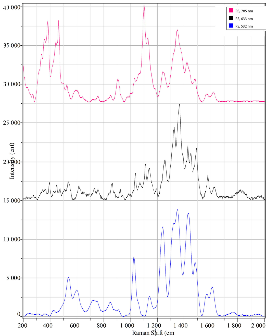
17. ábra: A kezeletlen pamutszárlól készült Raman-spektrumok. A piros spektrum a 785 nm-es lézerrel, a fekete a 633 nm-es lézerrel, a kék pedig az 532 nm-es lézerrel készült.
