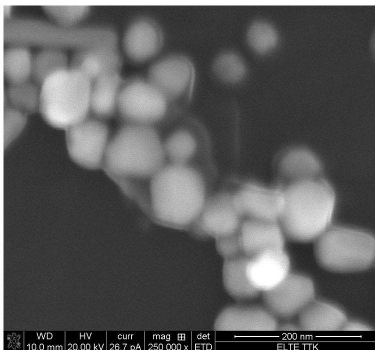
9. ábra: A csepp belsejének szennyeződésmentes része az ezüst részecskékkal és az azokat körülvevő burokkal. A szemcsék átlagos mérete 60 – 90 nm körüli érték.
