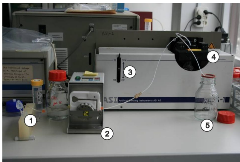
3.5. ábra. A mérőberendezés - ASI BIOS-1. – 1. Áramoltatott oldat, 2. perisztaltikus pumpa, 3. polarizátor, 4. küvetatartó, 5. a cellából távozó folyadék [13]
