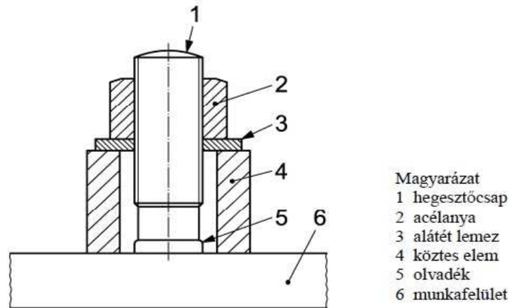
7. ábra Szakítóvizsgálat
