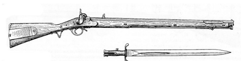
29. 1828 M kovás gyalogsági puska
