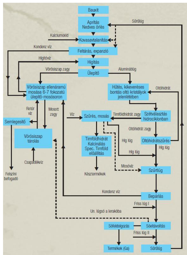
2. ábra: Az alumíniumtermelés folyamata 15
