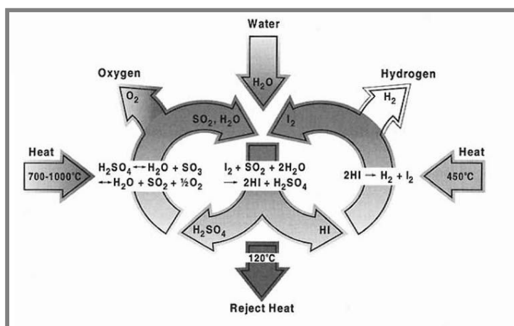
7. ábra: A többlépcsős termokémiai hidrogéntermelés folyamatábrája
