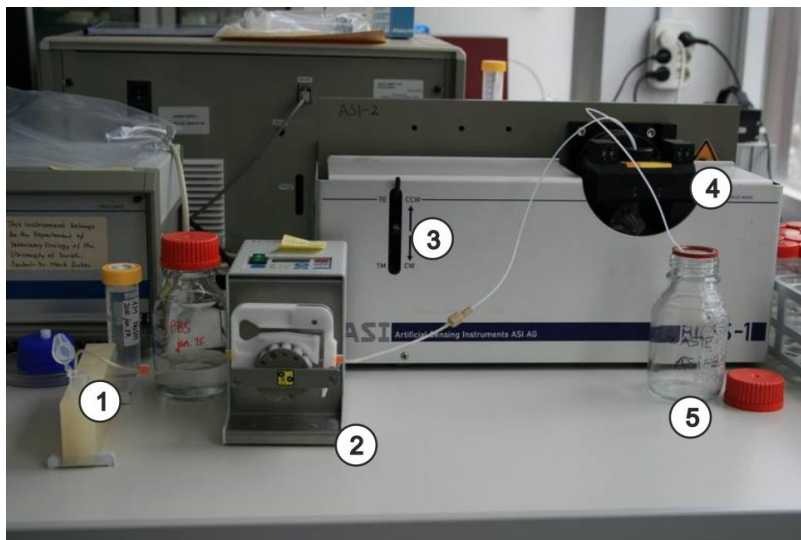
3.5. ábra. A mérőberendezés - ASI BIOS-1. – 1. Áramoltatott oldat, 2. perisztaltikus pumpa, 3. polarizátor, 4. küvet tartó, 5. a cellából távozó folyadék [13]
