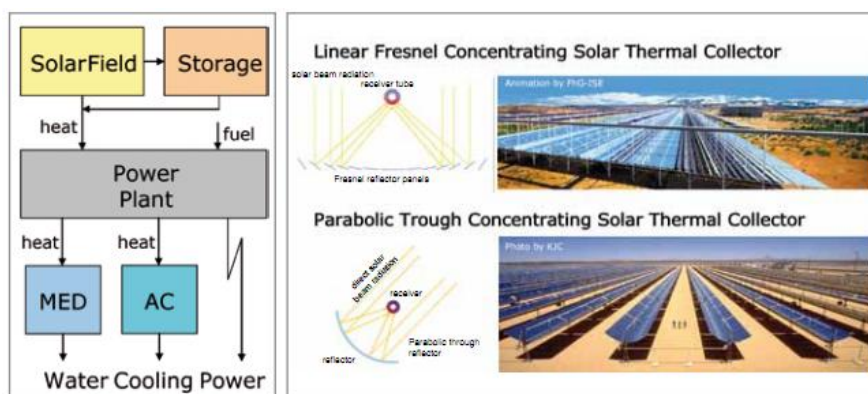
7. ábra A szolártermikus erőművek működési elve 26
