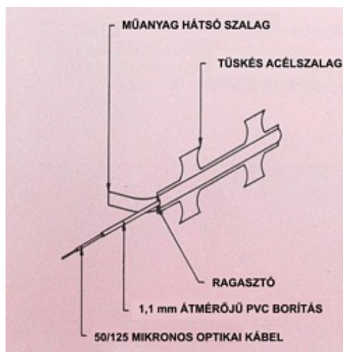
2. ábra: Az ún. NATO-drót szerkezete (forrás: http://oktel.hu/ , letöltve: 2012. 04. 12.)
