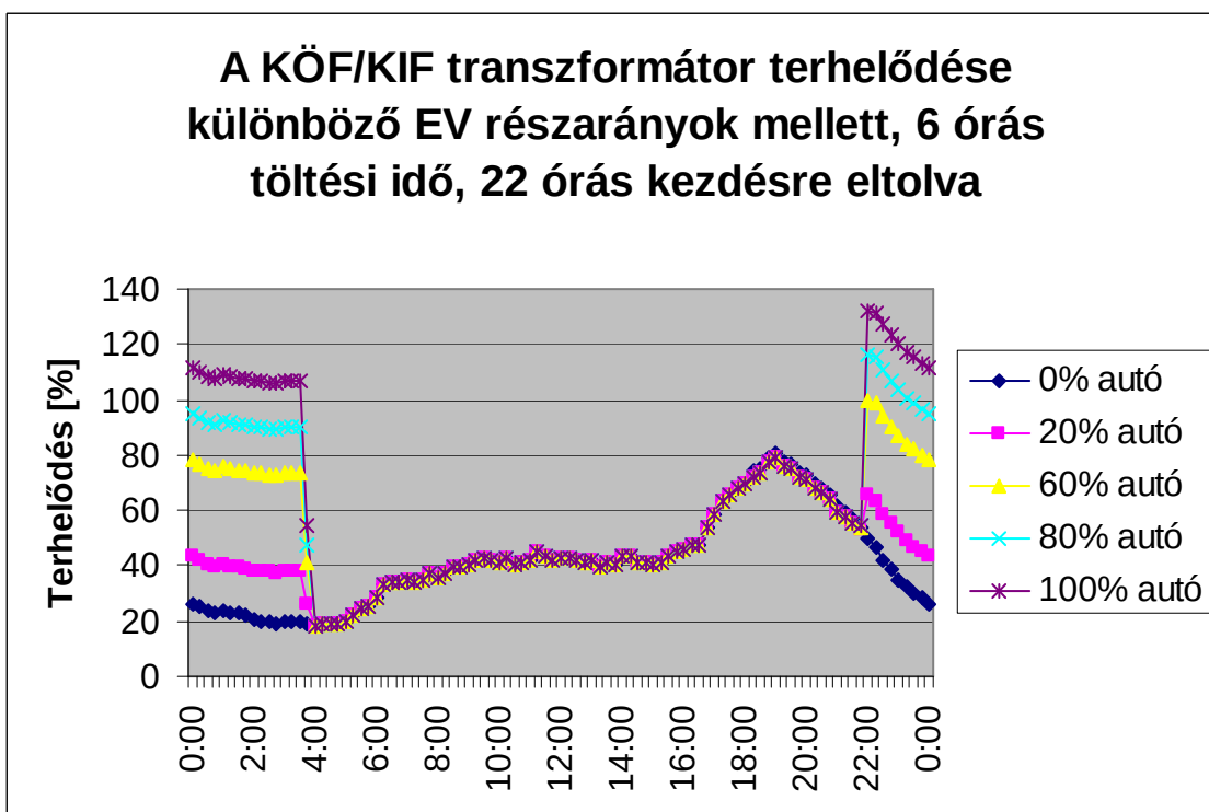
51. ábra: A KÖF/KIF transzformátor terhelődése 6 órás, 22 órára eltolva kezdésű töltés esetén
