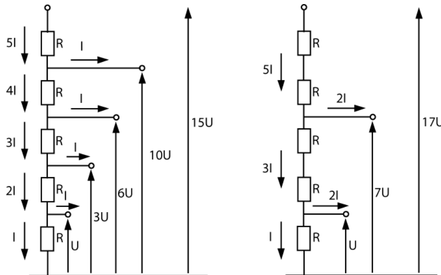
33. ábra: Annak szemléltetése, hogy a villamos autók térbeli eloszlása miatt befolyásolja az ellátó kábelben fellépő feszültségesést
