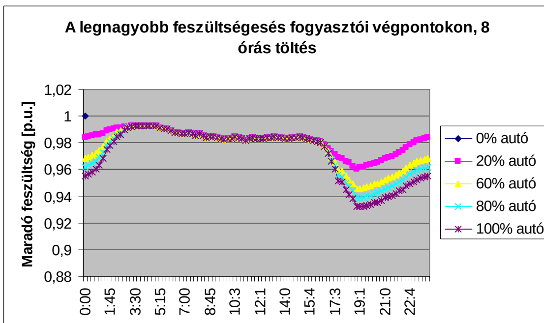
57. ábra: A legnagyobb feszültségesés fogyasztói végpontokon, 8 órás, eltolás nélküli töltés esetén
