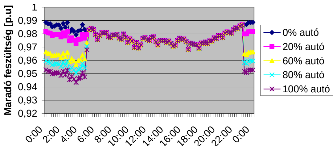
48. ábra: A legnagyobb feszültségesés fogyasztói végponton, 6 órás, 23 órára eltolt kezdésű töltés esetén
