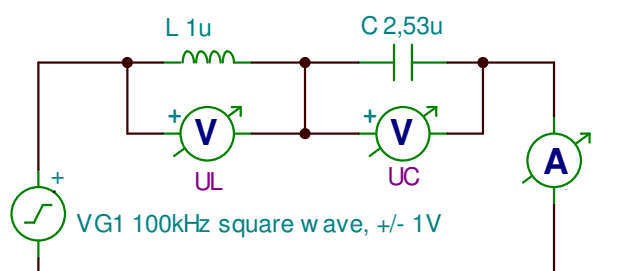
1. ábra: négyszög feszültséggel gerjesztett, 100 kHz sajátfrekvenciájú LC kör
