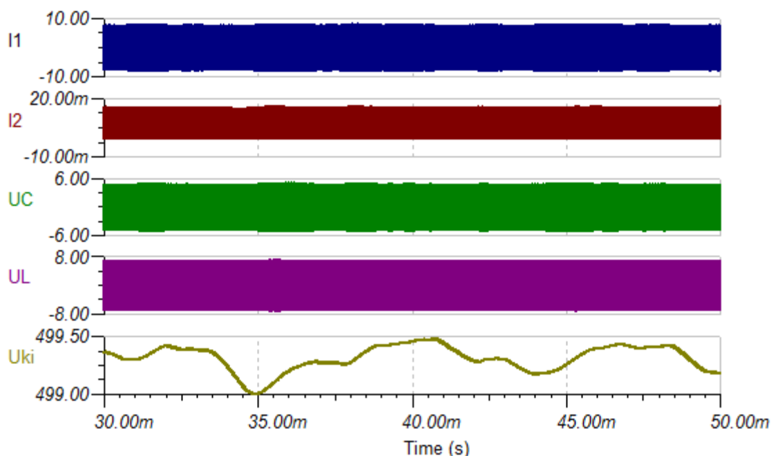
8. ábra: TINA szimuláció: a terhelt tápegység állandósult állapotban. R_t = 50 \text{ k}\Omega , C_{ki} = 1 \mu\text{F}
