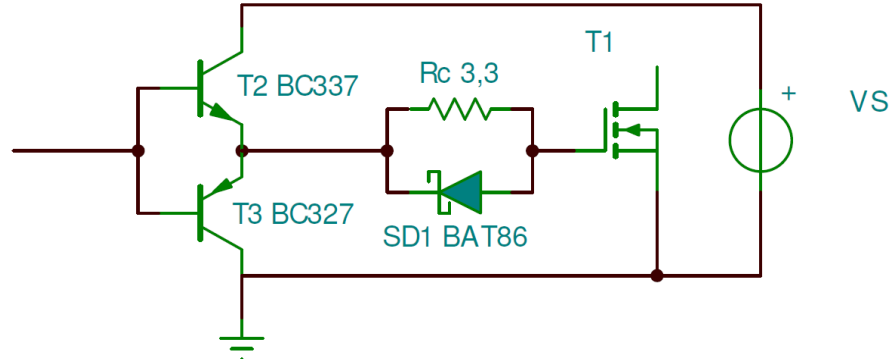
20. ábra: MOSFET gate meghajtó áramkör
