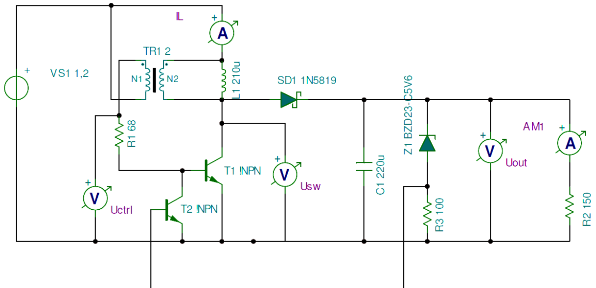
21. ábra: "Joule thief" önregző BOOST konverter kapcsolási rajza
