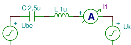
6. ábra: a sajátfrekvenciáján gerjesztett soros tápegység modellje
