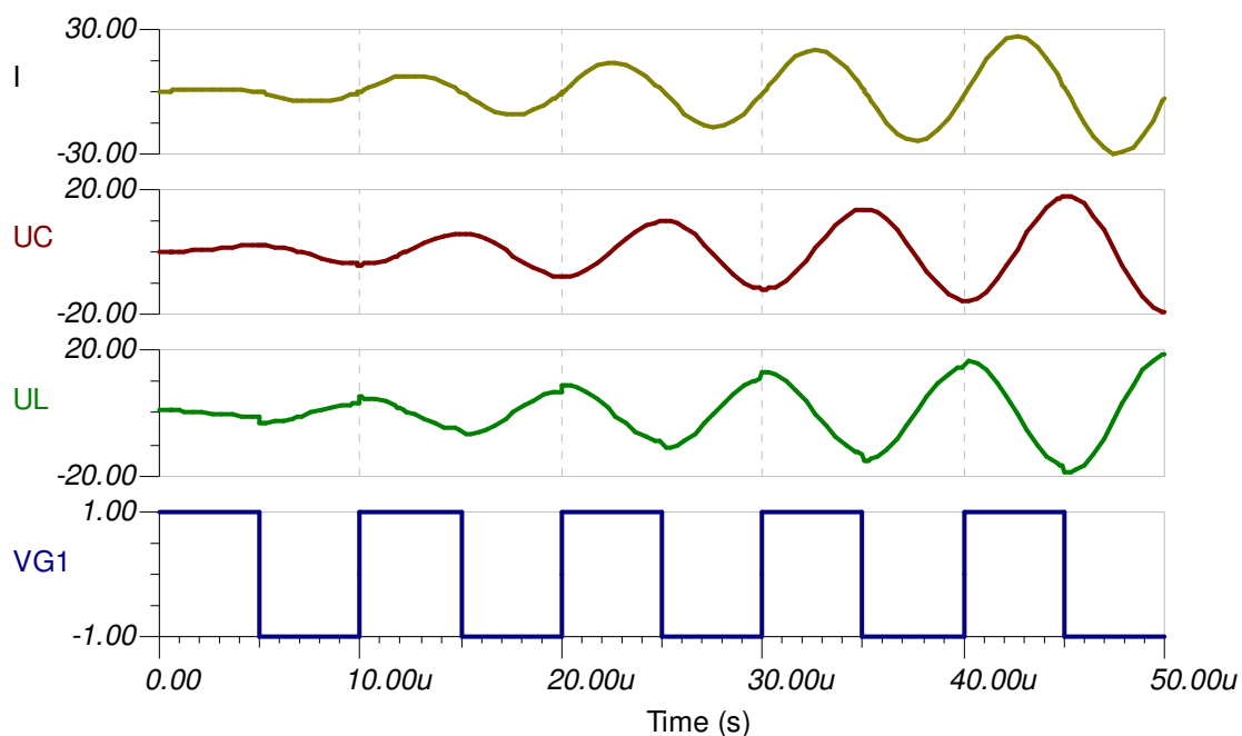
3. ábra: az 1. ábralátható LC kör időtartománybeli szimulációja TINA programmal
