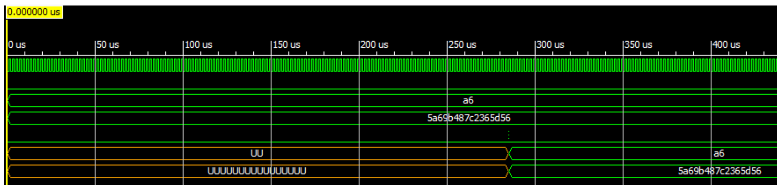
A bemenetre a FrameInV magas értéke mellett beállítottam egy fejléctet (HeaderIn) és egy csomagot (PacketIn), majd figyeltem a FrameOutV magas értéke mellett megjelenő fejléctet és csomagot. Azt vártam, hogy ugyanazt az adatot kapom vissza, mint amit megadtam. A keretezőt rákötöttem az USRT adó és vevő modulokra, azokat pedig összekötöttem. Ez az összeköttetés a normális működés során nem található meg, ha a WCLOCK felől nézzük, ide kapcsolódik a monitorozó kártya USRT adó és vevő modulja. Az eredményt a 34. ábra mutatja.
