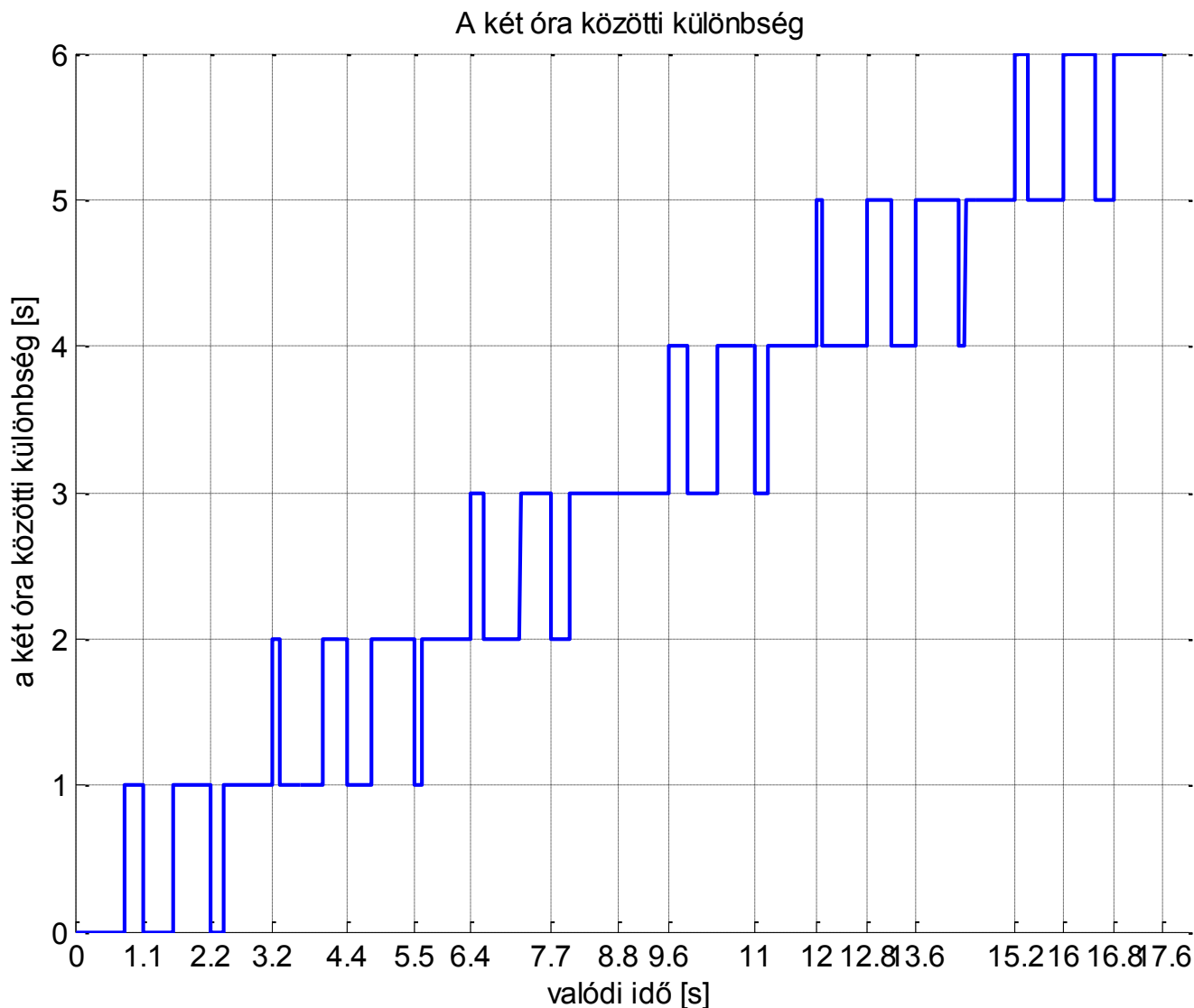
9. ábra: A 0,8 s és az 1,1 s periódusidejű órák különbsége
