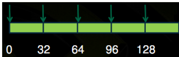
13. ÁBRA UNCOALESCED GLOBÁLIS MEMÓRIA OLVASÁS[4]
