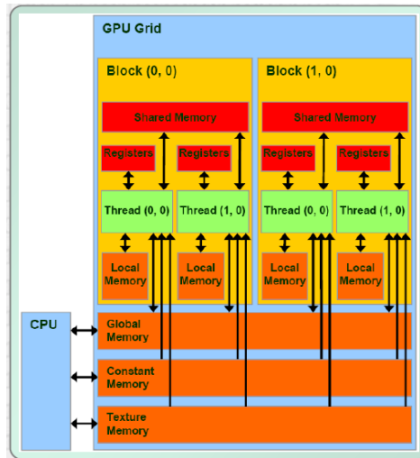
6. ÁBRA: CUDA ARCHITEKTÚRA [6]
