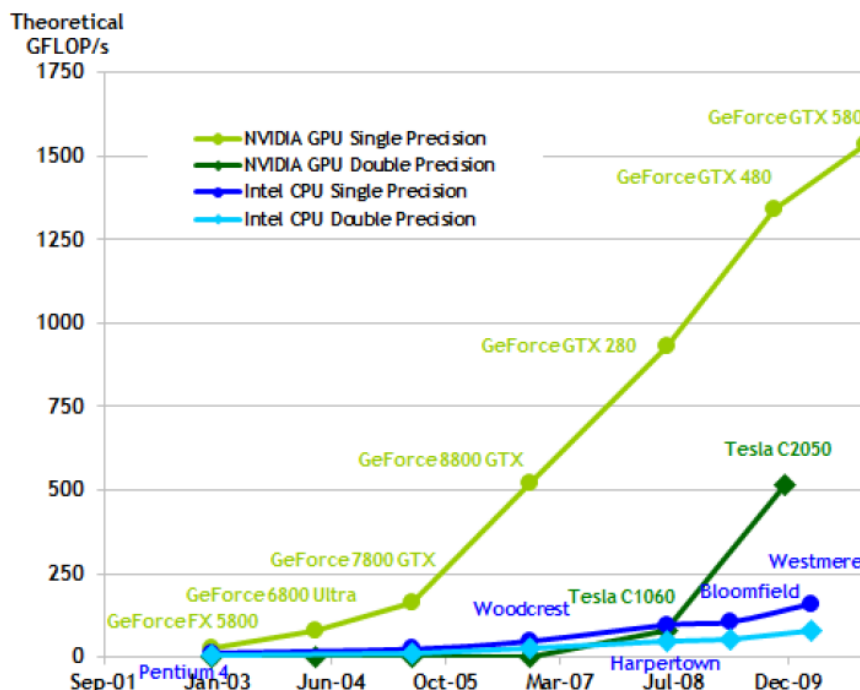
1. ÁBRA GPU-CPU LEBEGŐPONTOS SZÁMÍTÁSI KAPACITÁSÁNAK ÖSSZEHASONLÍTÁSA[4]
