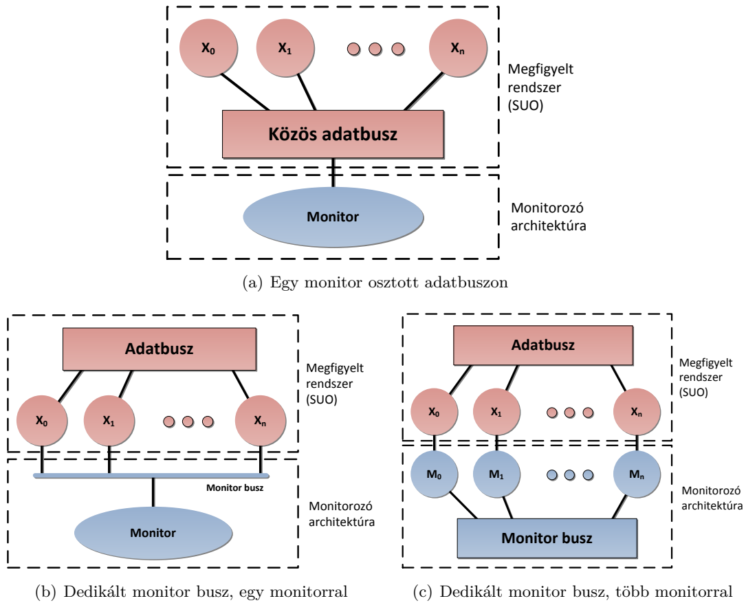
3.1. ábra. A [23]-ban ajánlott monitorozó architektúrák
