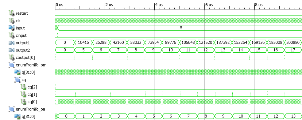
4.17. ábra. Ssum modul szimulációs hullámformája 10 us nagyságú intervallumban
