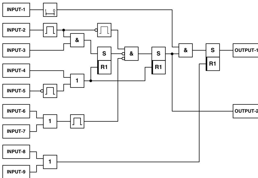
7.3. ábra. A PRISE-modell funkcionális blokkdiagramja [20]
